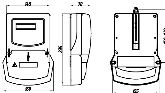
Рисунок А.2 – Тип корпуса Ш33
