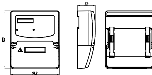
Рисунок А.1 – Тип корпуса Р32
