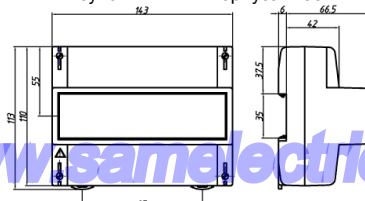
Рисунок А.3 – Тип корпуса Р31
