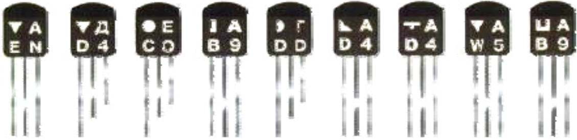
KT326AM 11.1994 г. KT3107DM 04.1993 г. KT503E 10.1992 г. KT681A 09.1991 г. KT502Г 12.1993 г. KT3157A 04.1993 г. KT3166A 04.1993 г. KT326 05.1998 г. KT3157A 09.1991 г.
