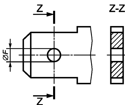
Рисунок К.5 — Размеры отверстий для фиксации
