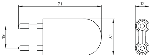
Рисунок 3 – Габаритные размеры средства контроля
