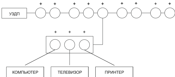
Рисунок 8 – Расширение зоны обслуживания удлинителем
