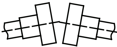
Рис. 2.6.1. Угловая несоосность
