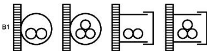
Провода/одножильные кабели в трубопроводах и коробах
