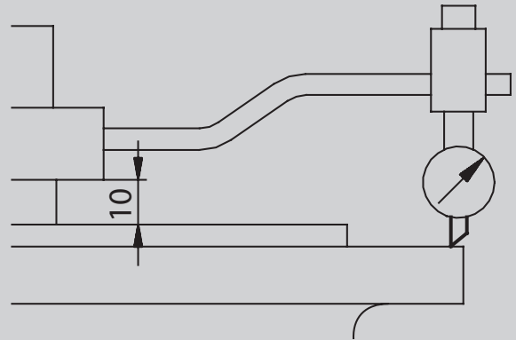
Перпендикулярность установочной поверхности фланца к валу
