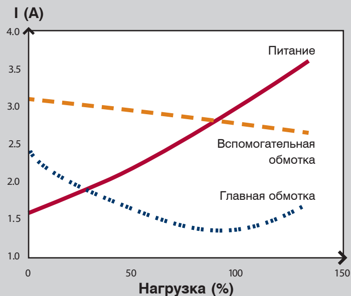
Пример хода токов в зависимости от нагрузки. Обратите внимание, что в фазах работы и пуска токи больше тока сети при нагрузке 0%.
