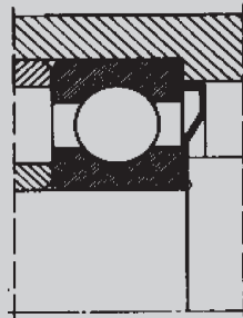
Установка подшипника с упругим металлическим уплотнением
