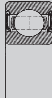
Шарикоподшипник с глубокими дорожками качения с резиновыми манжетами
