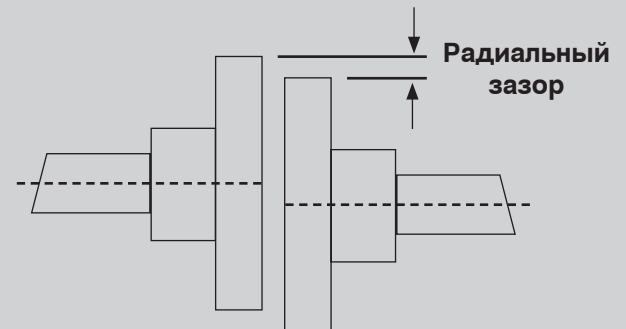
Радиальное согласование (концентричность) S_1
