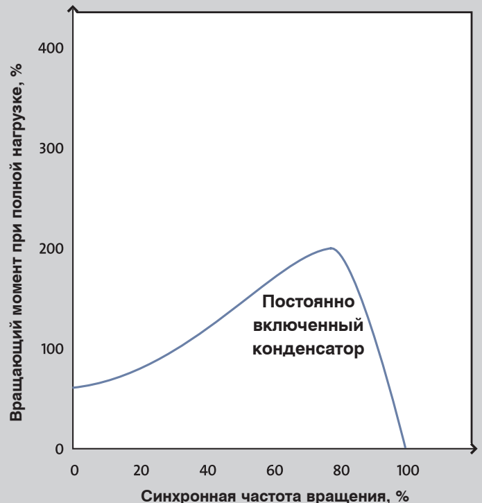
Электродвигатель PSC. Схема электрических соединений и характеристика пусковой момент/частота вращения
