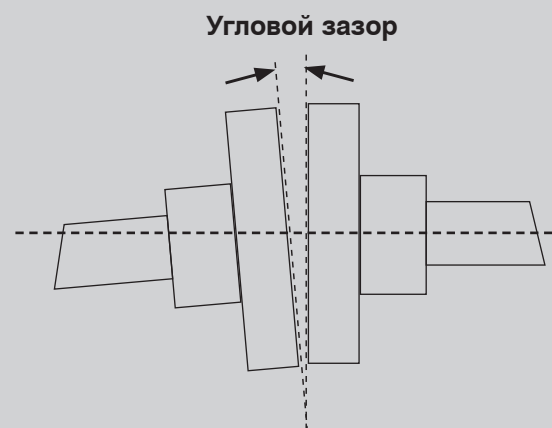
Угловое выравнивание
