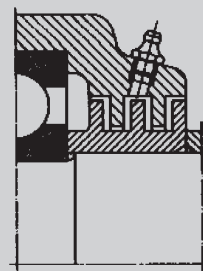
Лабиринтное уплотнение
