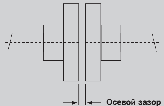
Согласование осей S_2
