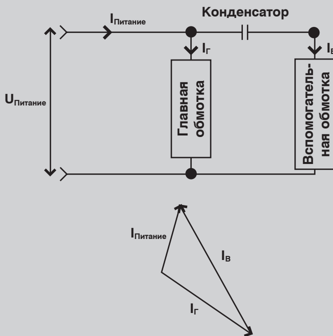
Пример асимметричного хода, когда ток в двух фазах больше, чем ток сети.
