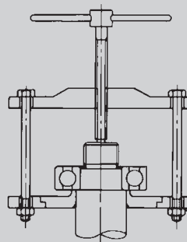
Выпрессовка подшипника
