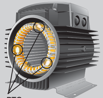
3 датчика ПТЦ; По одному на каждой фазе
