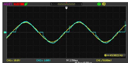
Рисунок 50 Форма тока с последовательным дуговым пробоем
