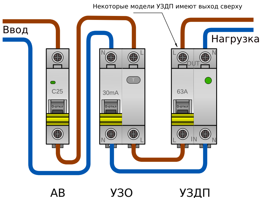
Рисунок 60 Схема включения УЗДП. Установка УЗО не обязательна. Внимательно изучите документацию, УЗДП могут иметь ввод как снизу, так и сверху. Фазировка УЗДП и УЗО обычно обозначена на корпусе.
