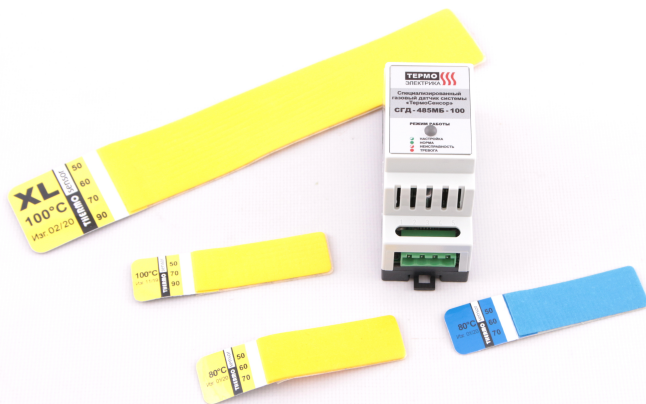
Рисунок 69 Газовыделяющие наклейки системы "термосенсор" с датчиком газа. Корпус датчика – обычный DIN-модуль на рейку.
