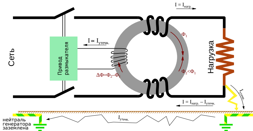
Рисунок 39 Принцип работы трансформатора токов современного УЗО
