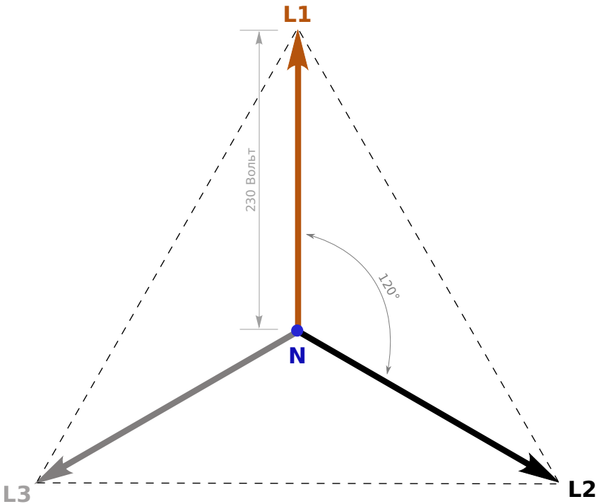
Рисунок 77 Векторная диаграмма.
