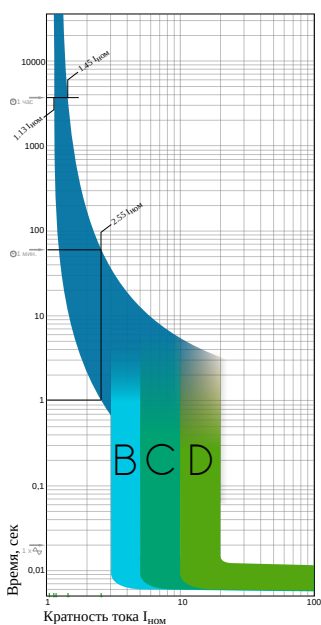
Рисунок 22 Времятоковые характеристики автоматических выключателей с типами электромагнитных расцепителей В, С и D
