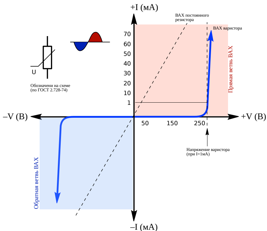
Рисунок 94 Вольт-амперная характеристика (VAX) варистора
