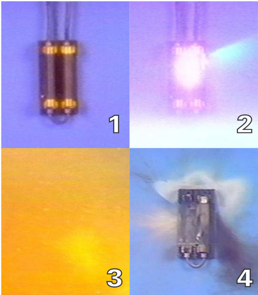
Рисунок 7 Кадры взрыва корпуса предохранителя от тока короткого замыкания свыше отключающей способности устройства. Иллюстрация из книги BUSSMANN Fuseology, стр 15.
