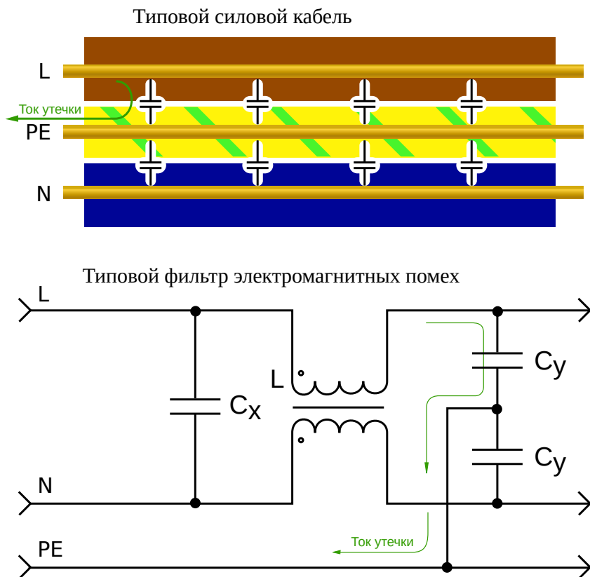
Рисунок 44 Пути утечки тока в PE проводник в исправном состоянии. Сверху показана паразитная ёмкость между проводниками в кабеле. Внизу изображена схема типового фильтра электромагнитных помех, который содержит любое электронное устройство.
