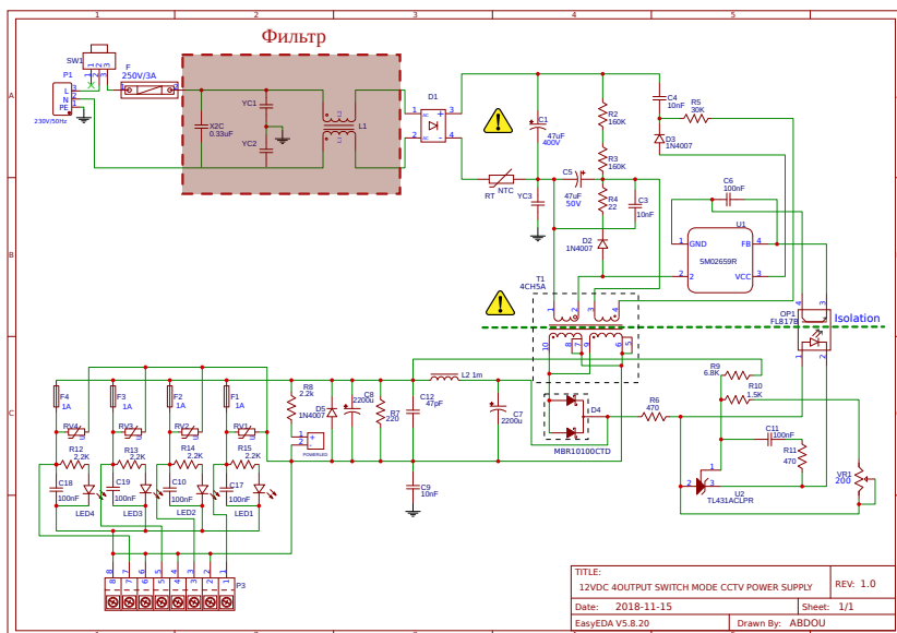
Рисунок 58 Схема импульсного блока питания с сайта oshwlab.com за авторством пользователя abduq. Фильтр я обвёл пунктиром.
