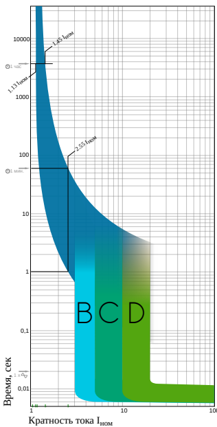
Рисунок 22 Времятоковые характеристики автоматических выключателей с типами электромагнитных расцепителей В, С и D
