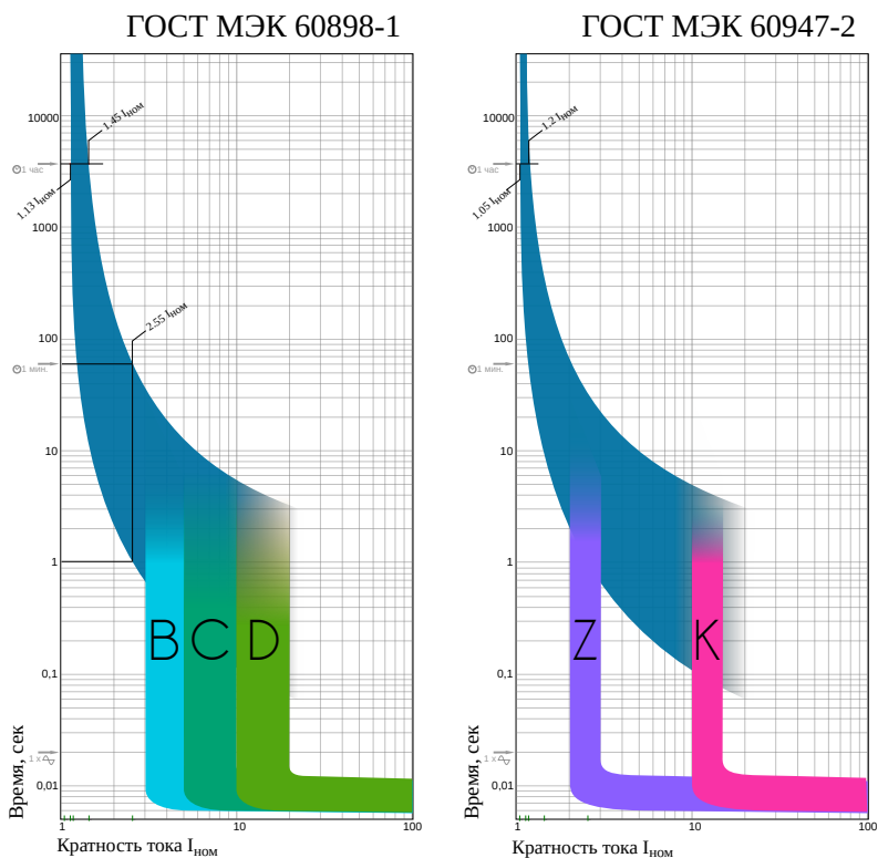
Рисунок 27 Времятоковые характеристики автоматических выключателей. Стандарт ГОСТ МЭК 60898-1 (слева) распространяется на бытовые автоматические выключатели, и типы электромагнитных расцепителей закреплены в стандарте. Справа времятоковые характеристики по ГОСТ МЭК 60947-2, который распространяется на промышленные автоматические выключатели. Типы электромагнитных расцепителей стандарт не описывает, производитель должен предоставить кривые времятоковых характеристик в документации. На графике нанесены кривые К и Z из документации компании АВВ.
