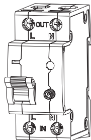
Рис.1. УСТРОЙСТВО
