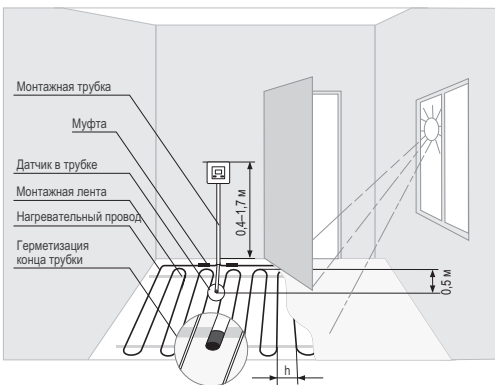
Рисунок 1. Монтаж терморегулятора и теплого пола
