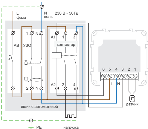
Схема 2. Подключение через магнитный пускатель
